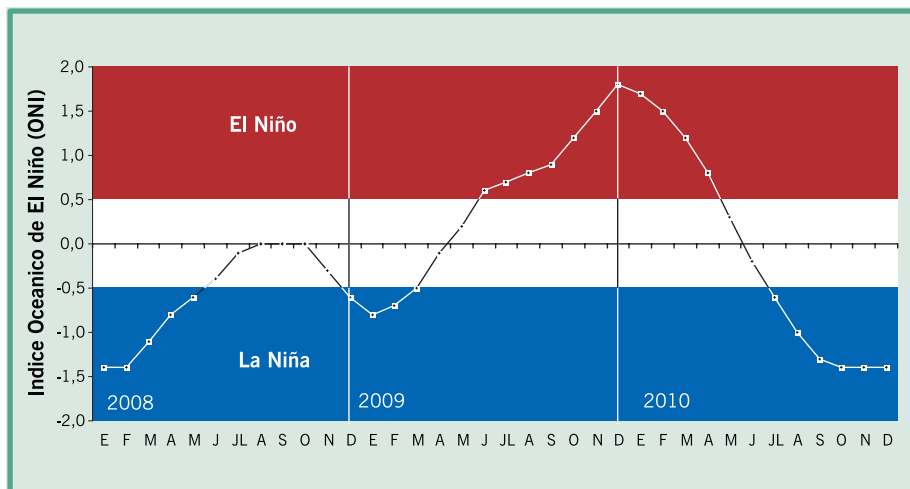
Figura 2. Distribución del Índice Oceánico de El Niño (ONI) para los años 2008, 2009 y 2010. La franja azul indica condiciones La Niña, la franja roja indica condiciones El Niño y la franja blanca indica condiciones neutras. Datos de tomados del Servicio Atmosférico y Oceánico de Los Estados Unidos (NOAA).
