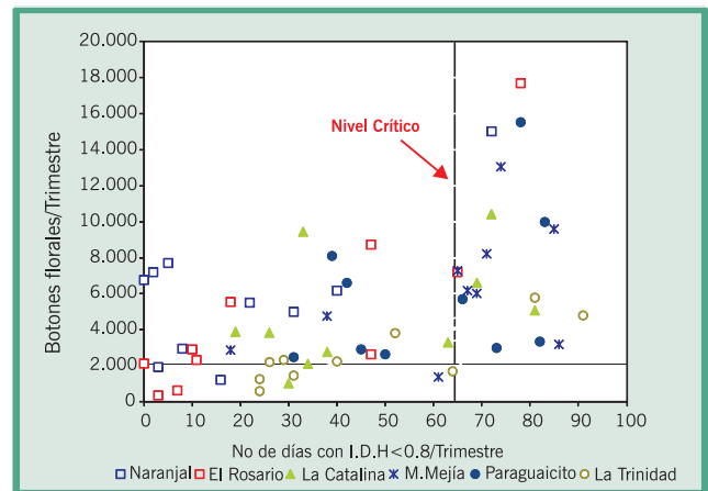
Figura 3. Relación entre el número de botones florales por trimestre y el número de días con déficit hídrico moderado.
