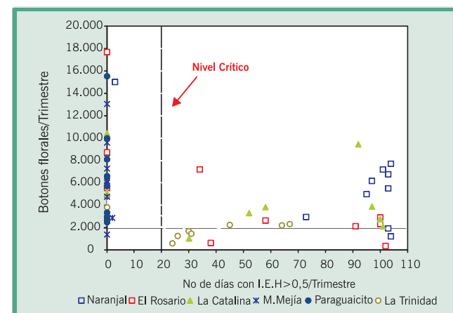
Figura 5. Relación entre el número de botones florales por trimestre y el número de días con exceso hídrico fuerte para café.
