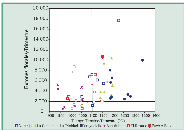
Figura 6. Relación entre el número de botones florales por trimestre y el tiempo térmico acumulado, calculado con una temperatura base de 10°C.
