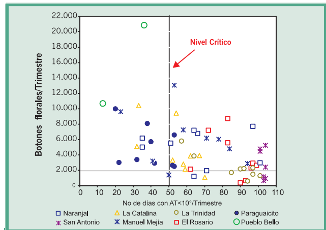
Figura 7. Relación entre la amplitud térmica ( AT = T_{max} - T_{min} ) y el número de botones florales por trimestre en café.
