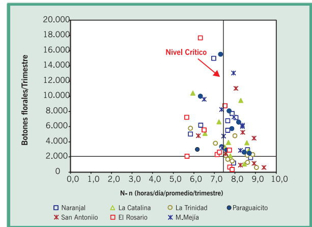
Figura 9. Relación entre el déficit de brillo solar promedio diario, por trimestre, y el número de botones florales en café.
