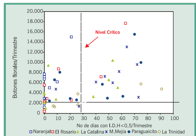
Figura 4. Relación entre el número de botones florales por trimestre y el número de días con déficit hídrico fuerte.
