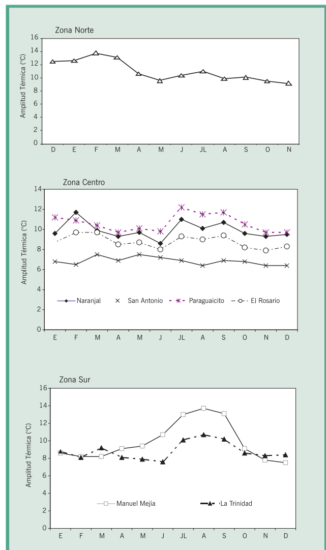
Figura 8. Distribución de la amplitud térmica en diferentes localidades de la zona cafetera Colombiana.
