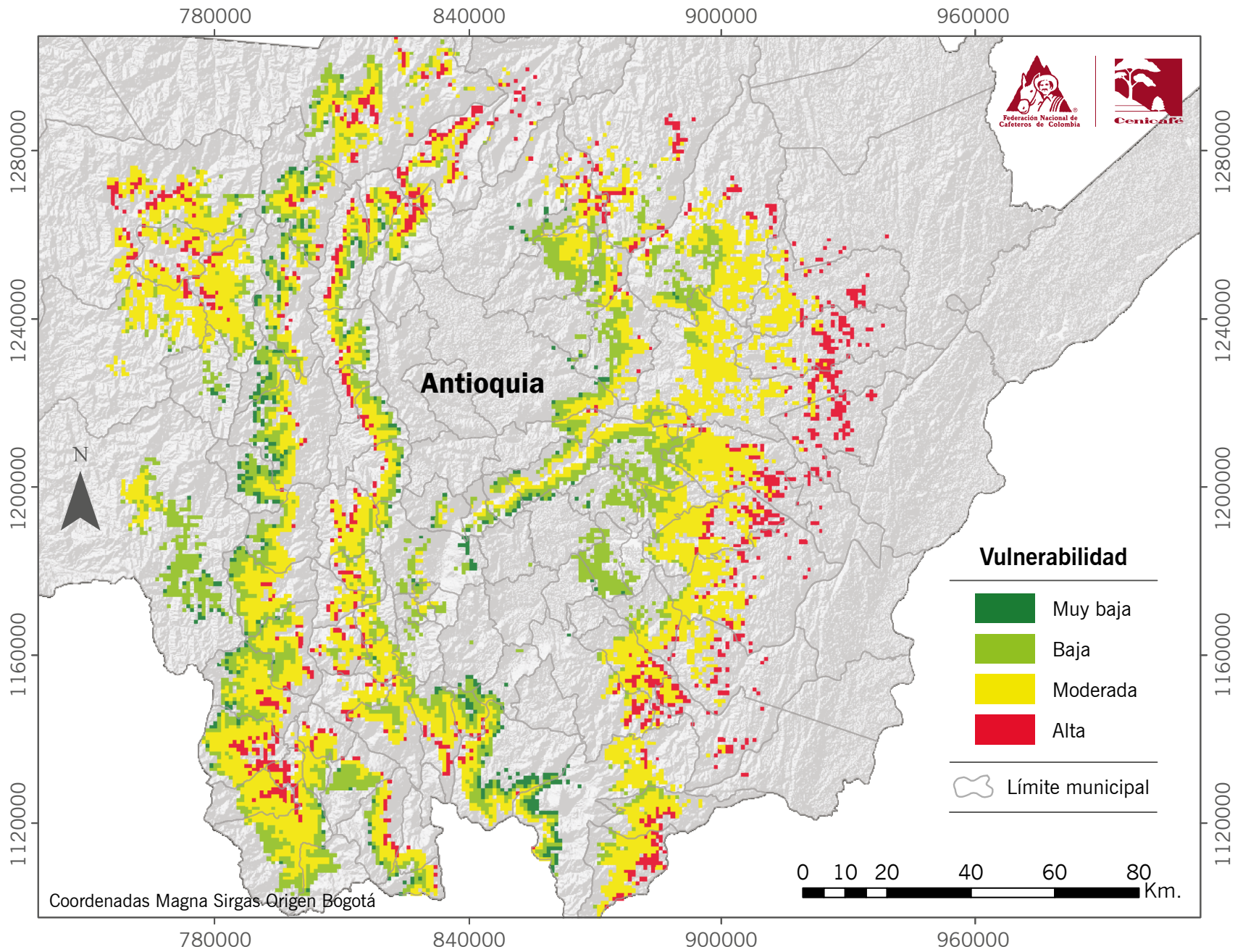
Figura 3. Mapa de vulnerabilidad de la zona cafetera de Antioquia a la broca del café en un año con escenario climático El Niño.
