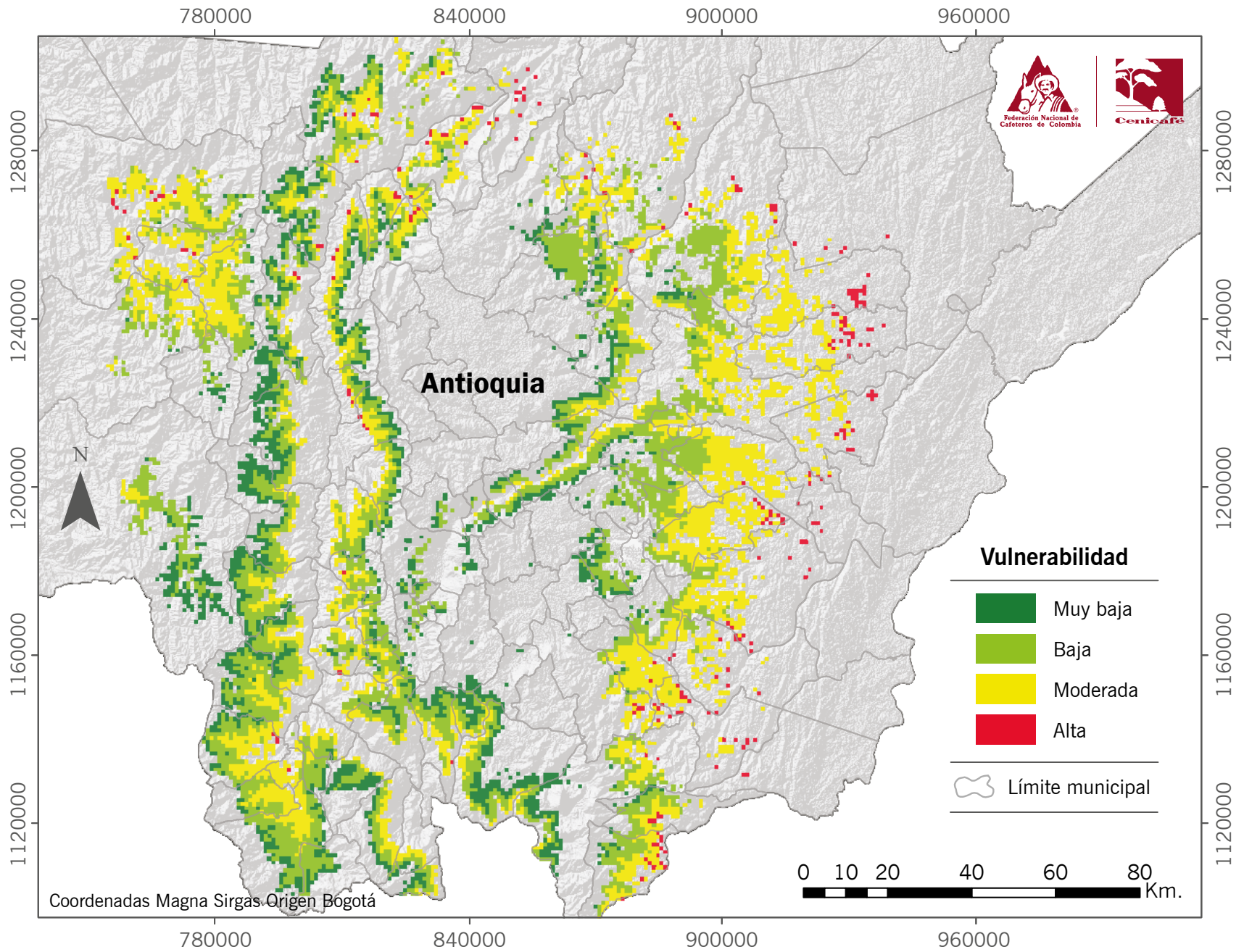
Figura 4. Mapa de vulnerabilidad de la zona cafetera de Antioquia a la broca del café en un año con escenario climático La Niña.
